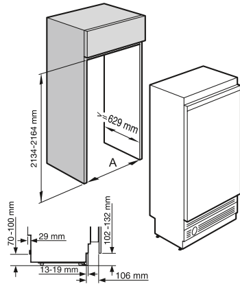
K1801Vi / KWT1601Vi
