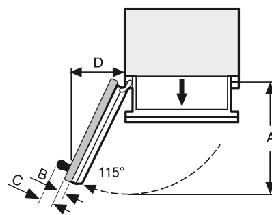
F1471Vi
