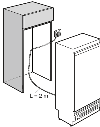
K1801Vi / KWT1601Vi
