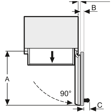
K1801Vi
